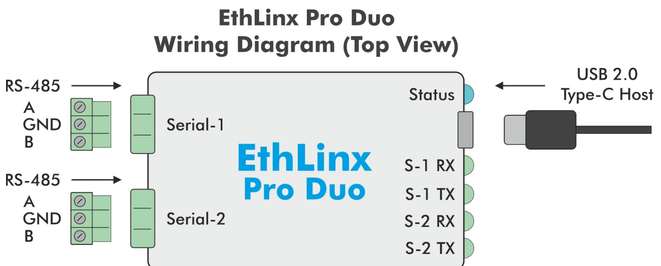
Abbildung 1: Grundlegender Schaltplan mit seriellen Anschlüssen und LED-Beschreibung, EthLinx Pro Duo
