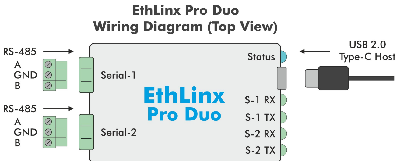
Image 1 : Schéma de câblage de base avec connexions série et description des LED, EthLinx Pro Duo
