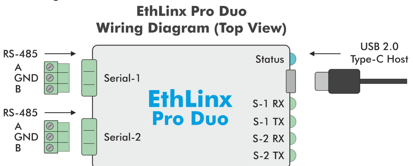
Afbeelding 1: Basis bedradingschema met seriële aansluitingen en LED-beschrijving, EthLinx Pro Duo
