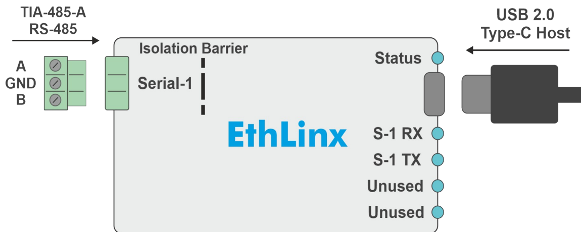
Imagen 1: Diagrama de cableado básico con conexiones serie y descripción de los LED, EthLinx
