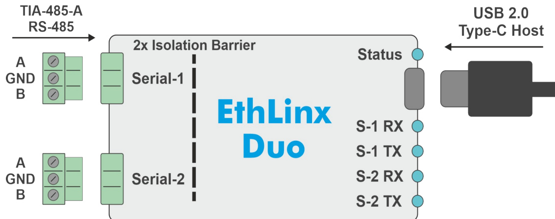
Imagen 2: Diagrama de cableado básico con conexiones serie y descripción de los LED, EthLinx Duo
