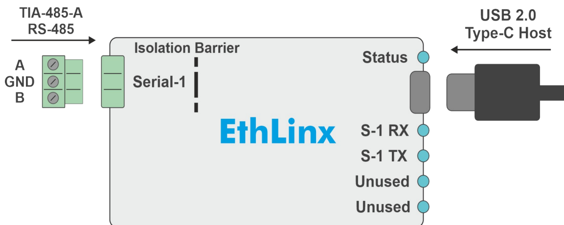
Image 1 : Schéma de câblage de base avec connexions série et description des LED, EthLinx
