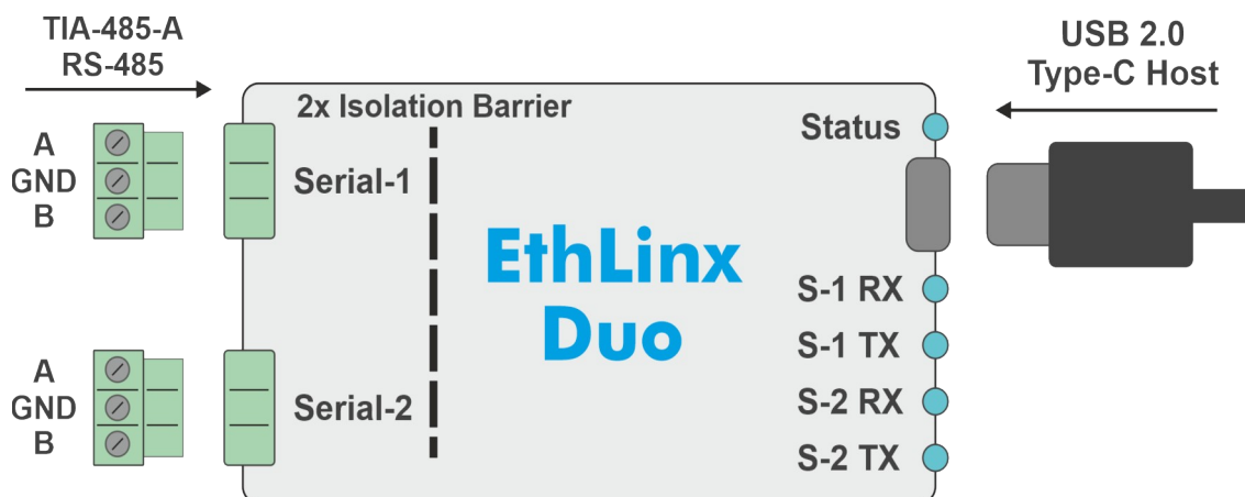
Image 2 : Schéma de câblage de base avec connexions série et description des LED, EthLinx Duo
