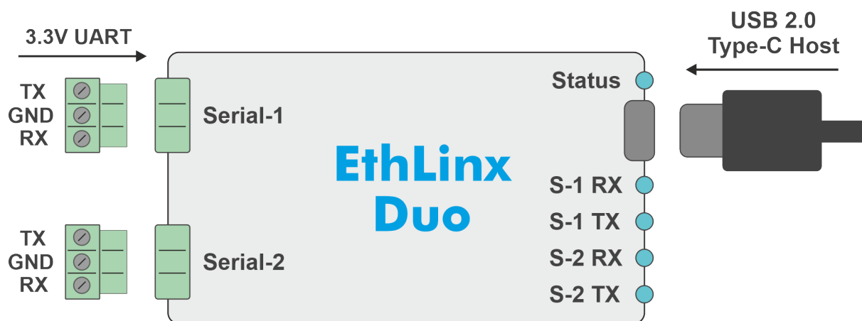
Abbildung 1: Grundlegender Schaltplan mit seriellen Anschlüssen und LED-Beschreibung, EthLinx Duo
