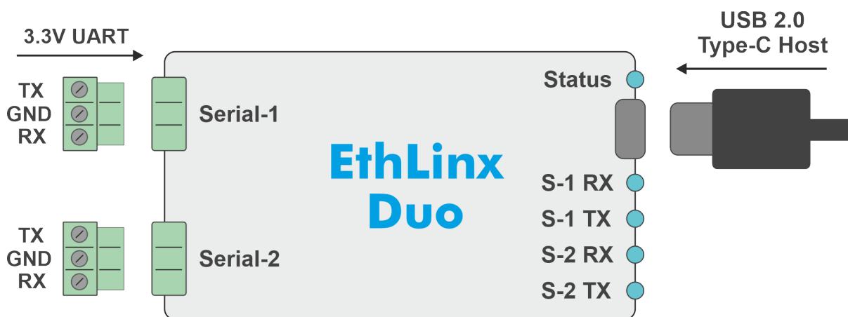
Image 1 : Schéma de câblage de base avec connexions série et description des LED, EthLinx Duo
